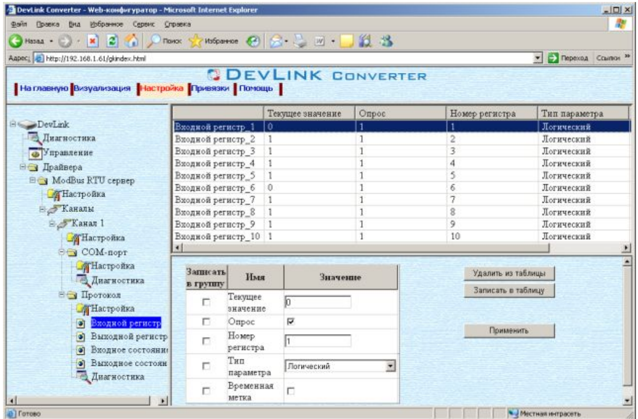
Рисунок 4.1 – Настройка. Входные регистры
