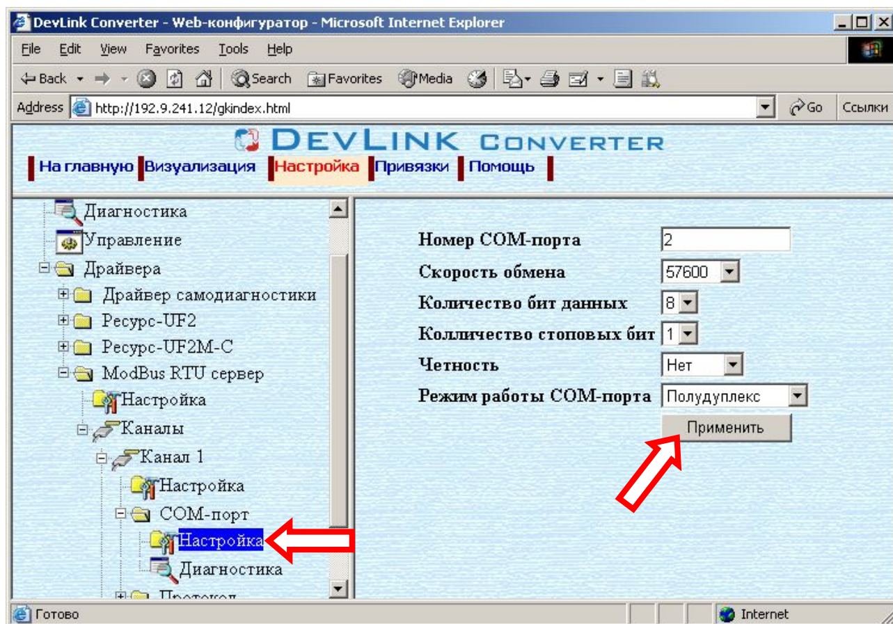
Рисунок 3.8 – Настройка COM-порта
